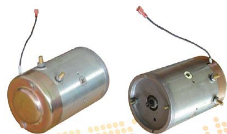
ZD1221 12V 2.0KW 2900RPM CW/顺时针 114MM
