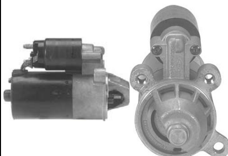
3217 2-1563-FD PMGR Ford 12V 1.4KW 10T
