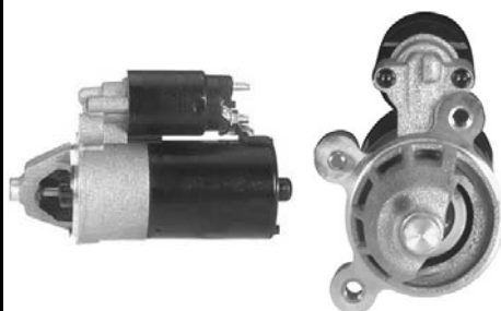
3267 2-1799-FD PMGR Ford 12V 1.4KW 12T
