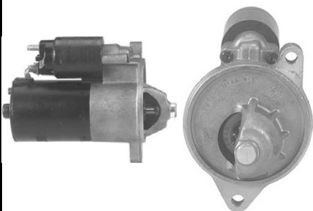
3223 2-1566-FD PMGR Ford 12V 1.4KW 10T
