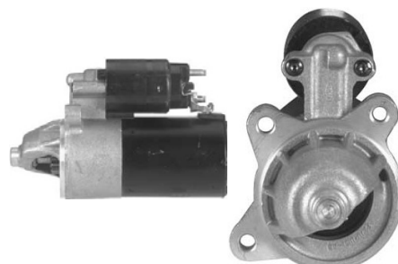
3221 2-1567-FD PMGR Ford 12V 1.4KW 10T
