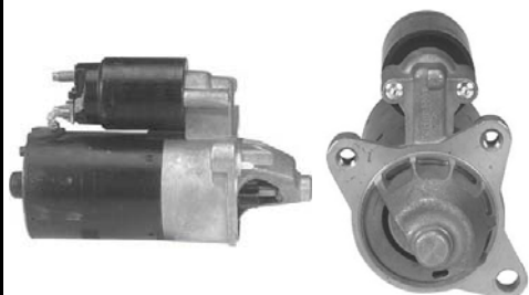
3214 2-1915-FD PMGR Ford 12V 1.4KW 9T
