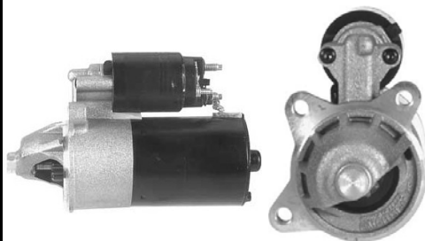
3263 2-1719-FD PMGR Ford 12V 22T
