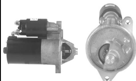
3223 2-1566-FD PMGR Ford 12V 1.4KW 10T
