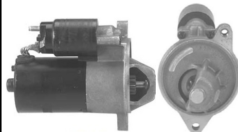
3221 2-1567-FD PMGR Ford 12V 1.4KW 10T
